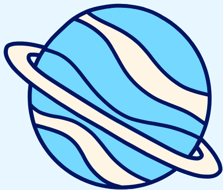
Urano
