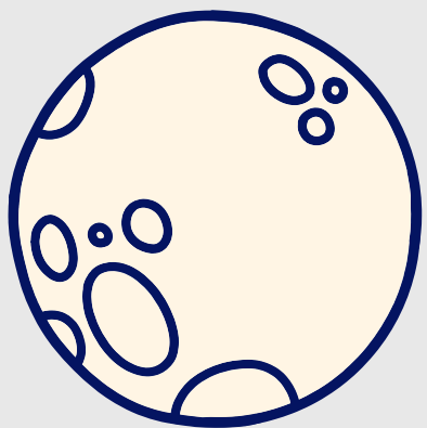
Lua
