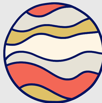
Júpiter
