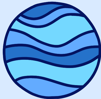
Netuno
