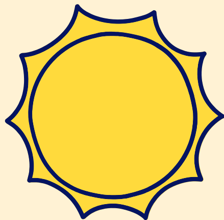
Sol
