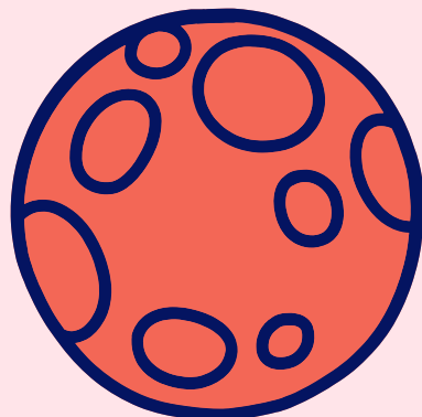
Marte
